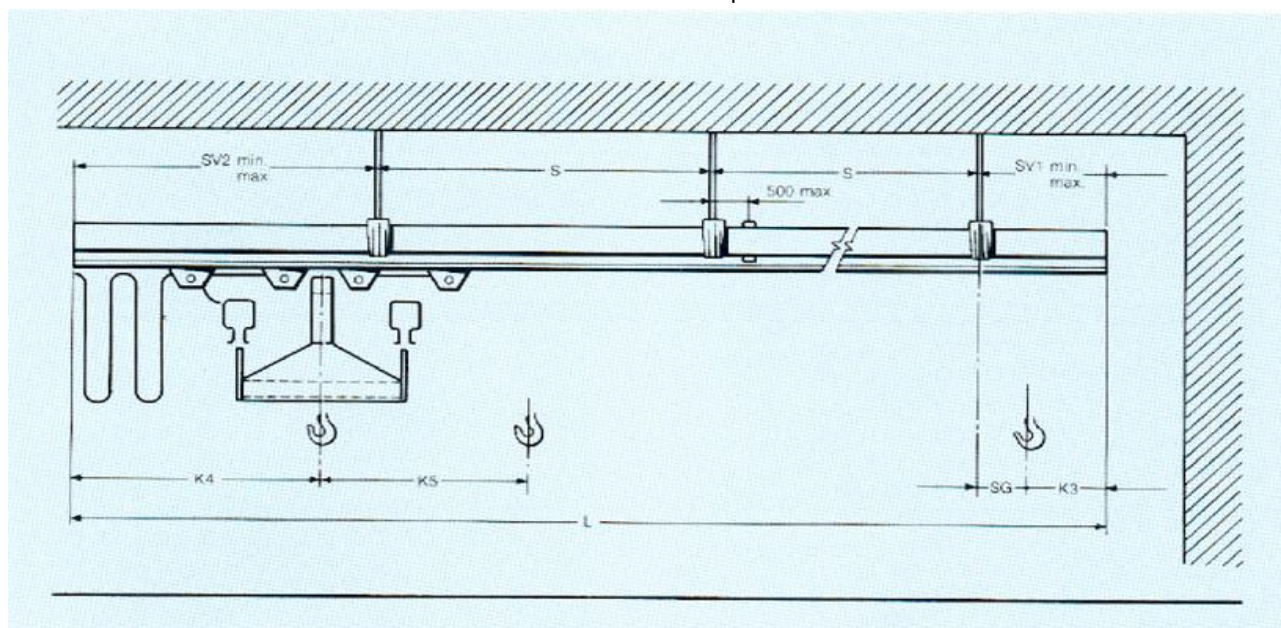
Dimensionnement des voies de course pour pont roulant bipoutre
