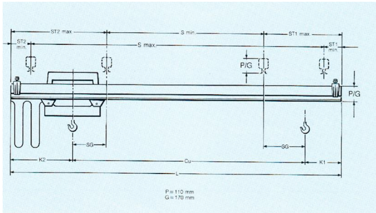
Dimensionnement pont roulant bipoutre
