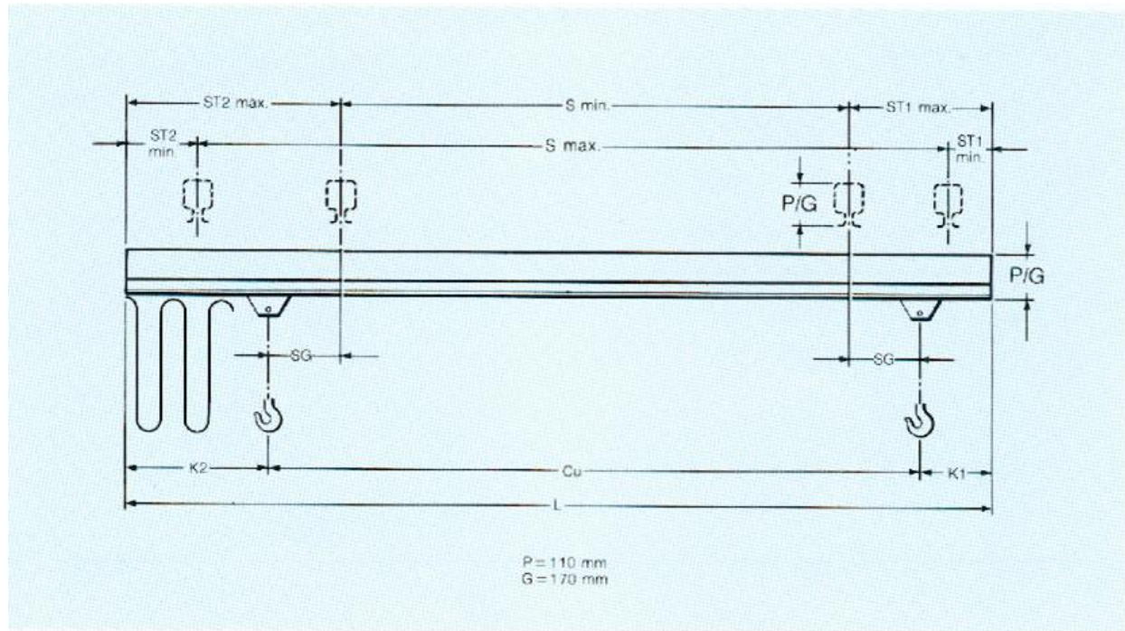
Dimensionnement pont roulant monopoutre
