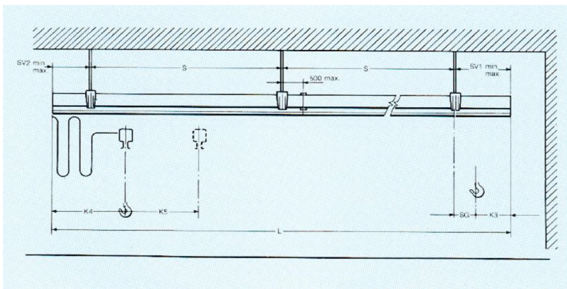
Dimensionnement des voies de course pour pont roulant monopoutre
